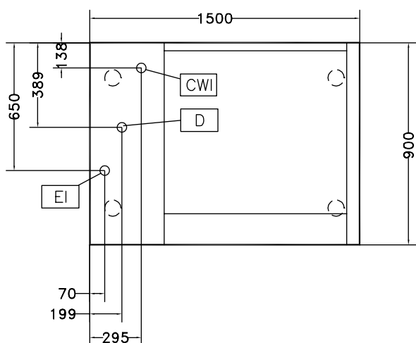
Felülnézet
